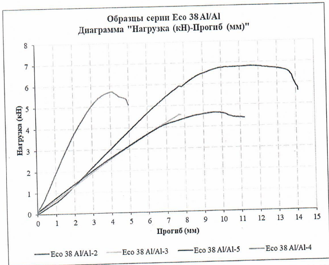
Рисунок 8. Диаграмма «Нагрузка (кН)-Прогиб (мм)» для образцов с серии Есо 38 АI/AI
