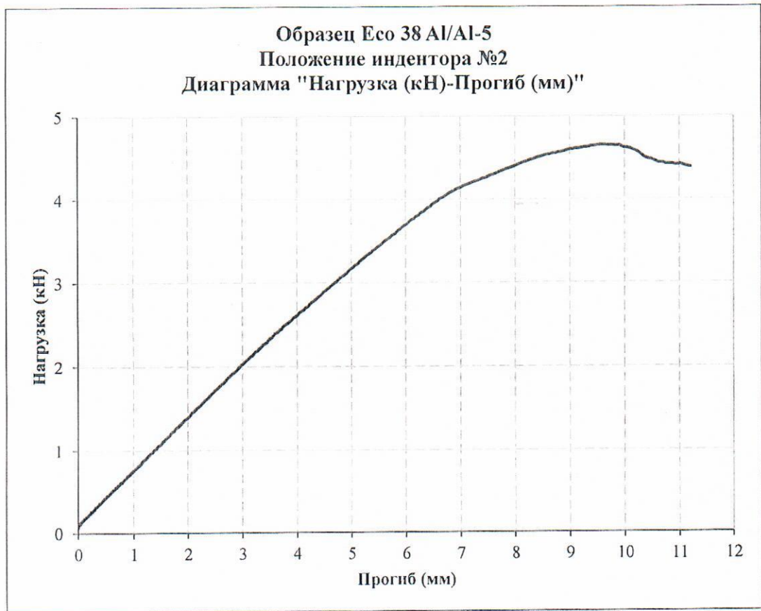
Рисунок 11. Диаграмма «Нагрузка (кН)-Прогиб (мм)» для образца 3
