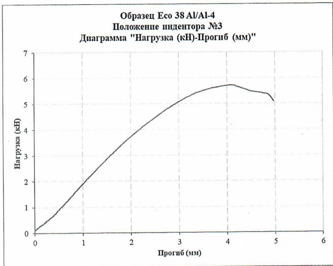
Рисунок 12. Диаграмма «Нагрузка (кН)-Прогиб (мм)» для образца 4
