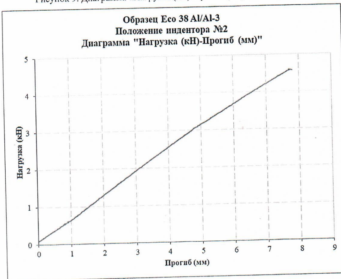
Рисунок 10. Диаграмма «Нагрузка (кН)-Прогиб (мм)» для образца 2
