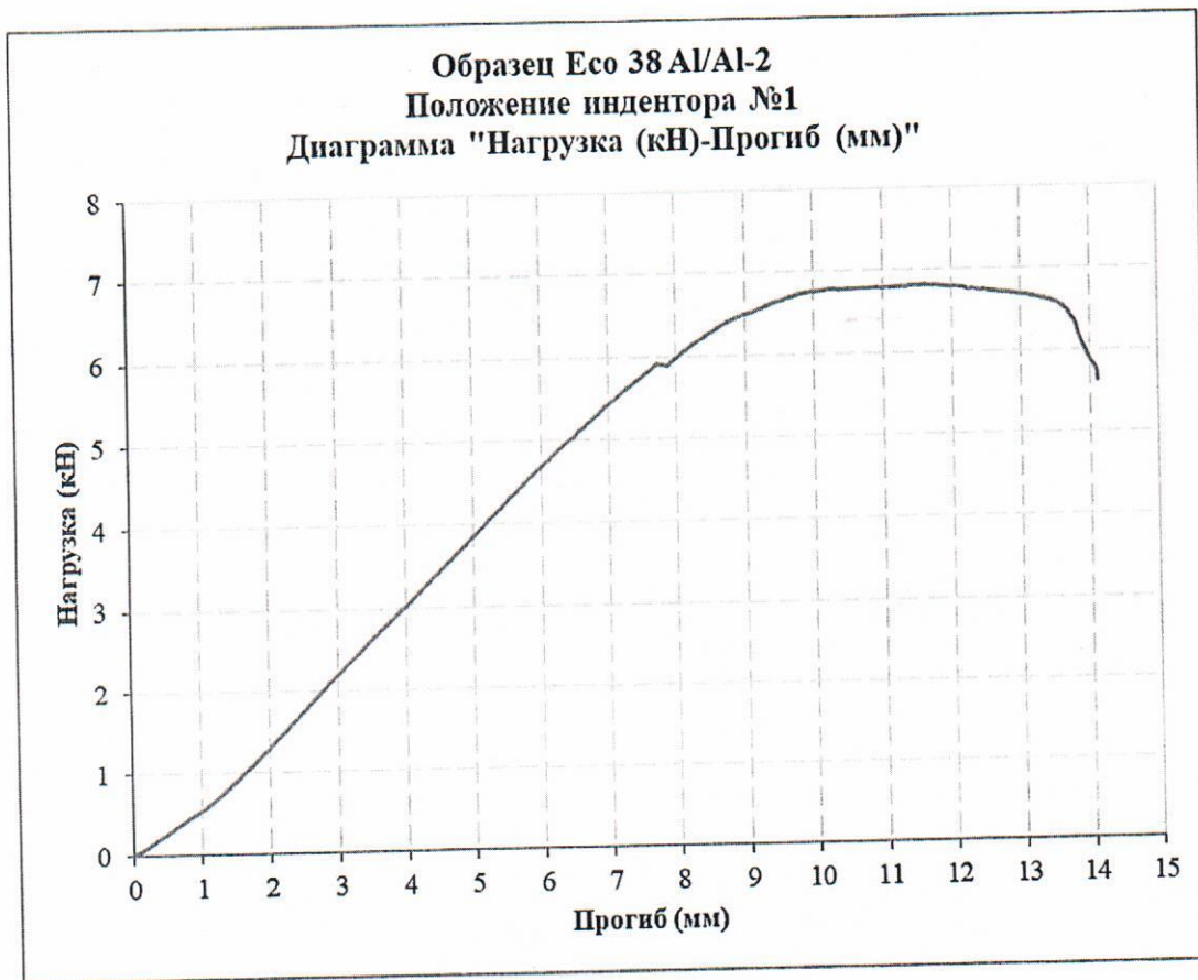
Рисунок 9. Диаграмма «Нагрузка (кН)-Прогиб (мм)» для образца 1
